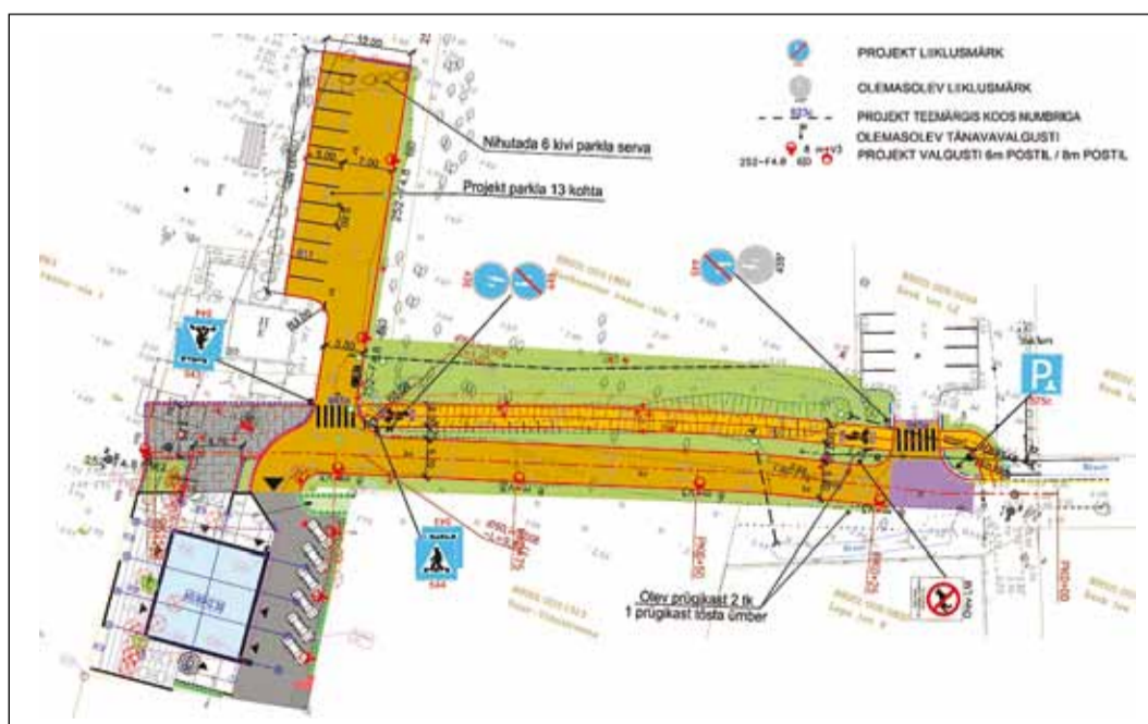
Kesk tee randa viiva lõigu rekonstrueerimisprojekt.
